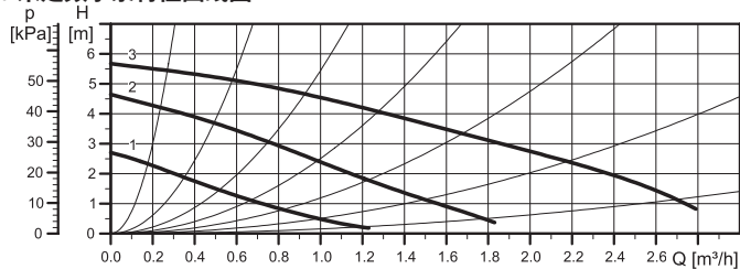
7 米定频水泵特性曲线图
